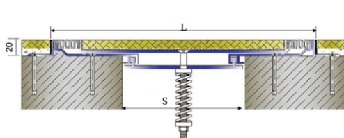
ДШ-ПС Н=20мм S=100-150мм
