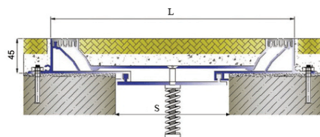
ДШ-ПС Н=45мм S=100-150мм
