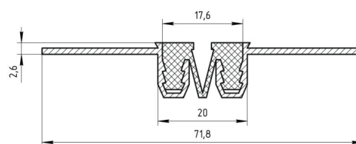
ДШ-СШ-20/2Г ( где Г – компенсатор гармошка)
